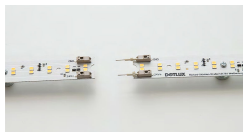
Mit Pin-Anschlüssen lassen sich die LED-Module in Reihe verbinden (inkl. Lösewerkzeug).
