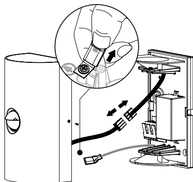
EASYbase für einfache Montage mit doppeltem Kabeleinlass.
